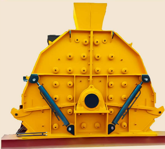
ماسه ساز دو طرفه 50-60 ton/h با الکتروموتور 75kw
