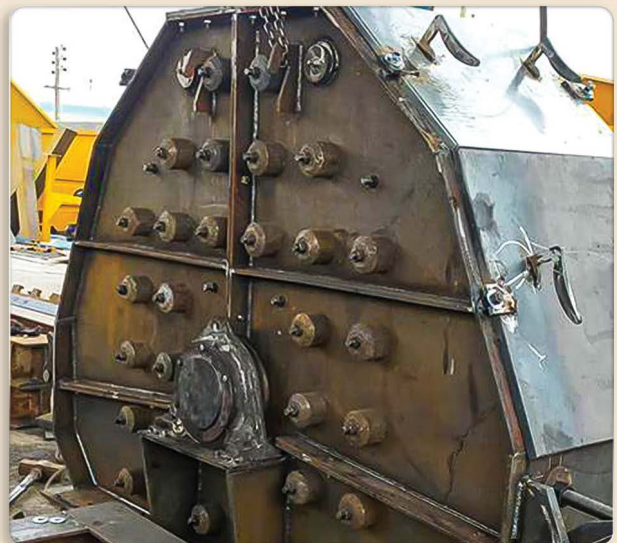
ماسه ساز دو طرفه 50-60 ton/h با الکتروموتور 75kw
